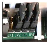
Jumper und Jumper-Steckplätze
