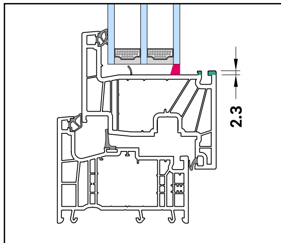
Μειωμένη βάση υαλοπίνακα για ευκολότερη κόλληση του τζαμιού.
