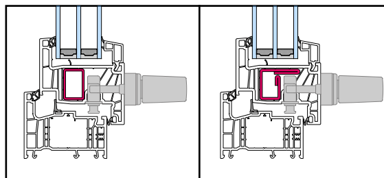
Δεν απαιτείται επεξεργασία του οπλισμού γενικής χρήσης (αριστερά) και του στατικού οπλισμού (δεξιά).
