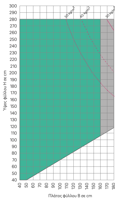
Φύλλο Z86 με σπλισμό 1358172 και συγκόλληση πλαισίου τζαμιού-φύλλου REHAU
