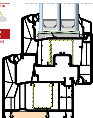
Sistema SYNEGO con junta central
