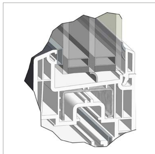
Konvektionsspærre
